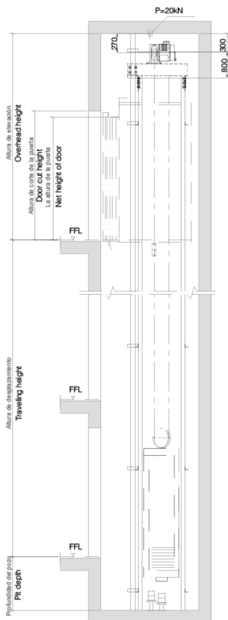
Hoistway elevation Elevación de la grúa
