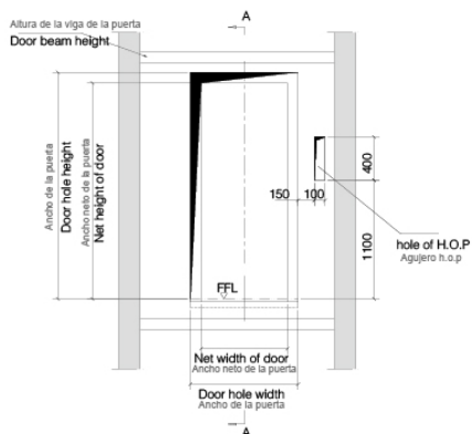
Front view of hoist way door Vista del plan de elevación
